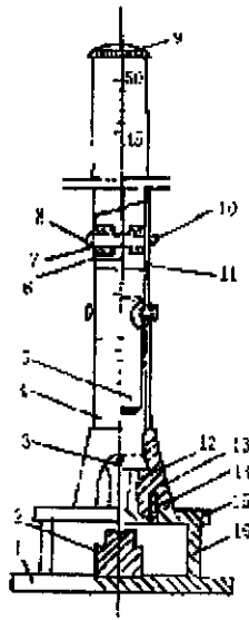
冲击试验器
